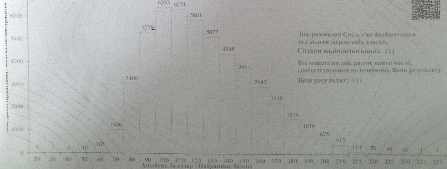
Негизги тест боюнча алган баллдын суммасына ылайык абитуриенттердин саны Количество абитуриентов в зависимости от суммы набранных баллов по основному тесту
